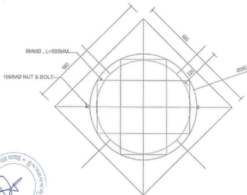
MANHOLE FRAME Scale : 1:10
